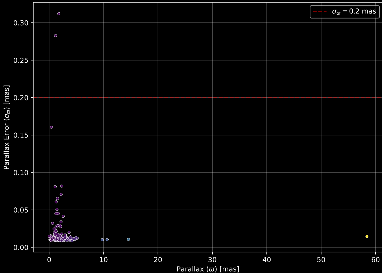
GALAH DR4 Field: [677] Parallax Quality (n= 283)
