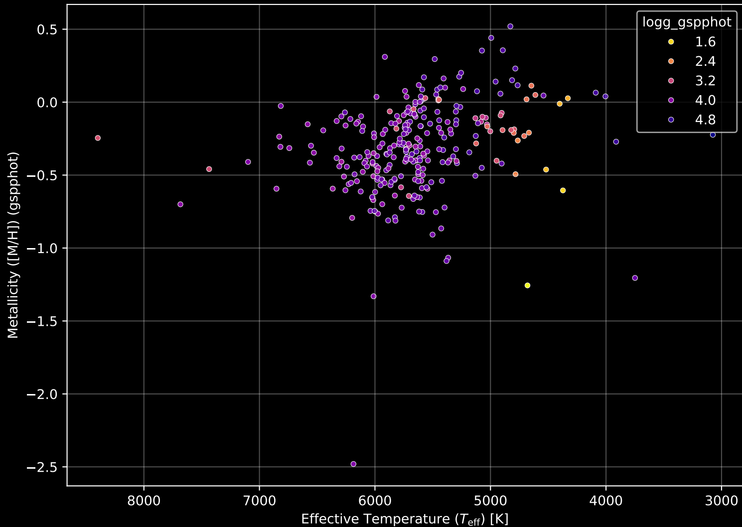
GALAH DR4 Field: [677] Stellar Population Parameters (n= 283)
